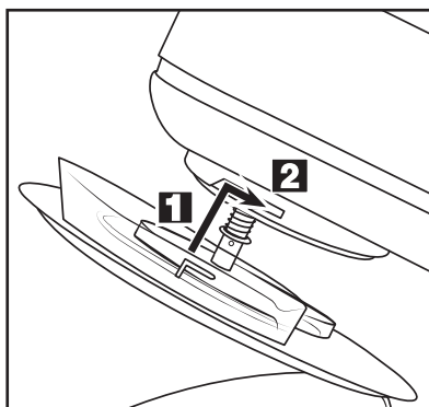
Fig. 1: montaje de la tapa 9
